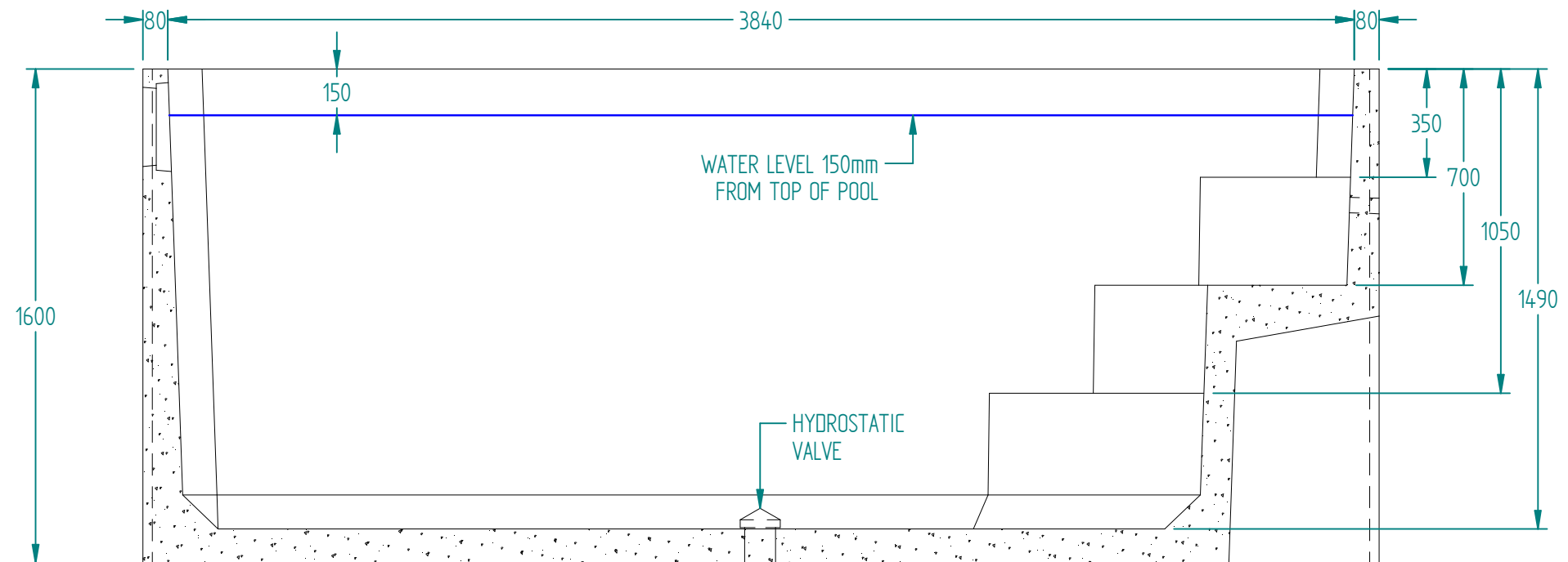
SECTION A-A 1:20
